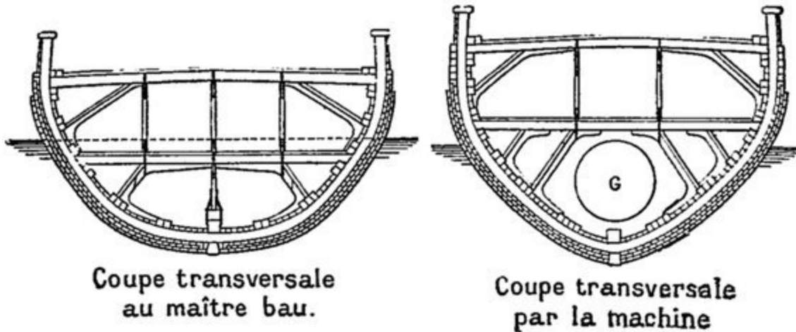
Coupe transversale au maître bau. Coupe transversale par la machine
